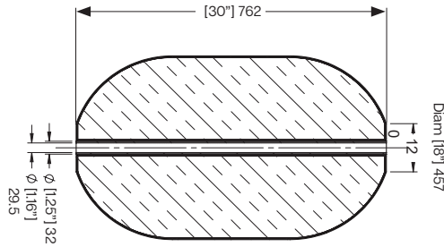
18" de Diámetro x 30" de Longitud Modelo: SL-BF-1830
