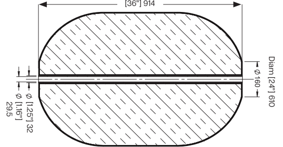
24" de Diámetro x 36" de Longitud Modelo: SL-BF-2436
