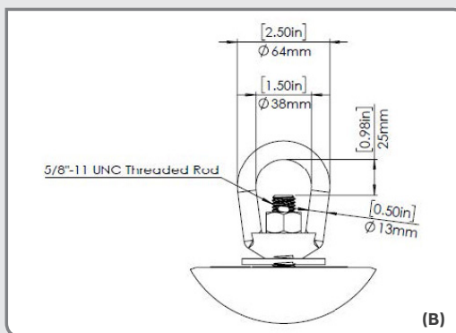
Ilustración (A) Dimensiones de Extremo de grillete en Flotador de barrera de 15" (SL-BF-15-S)
