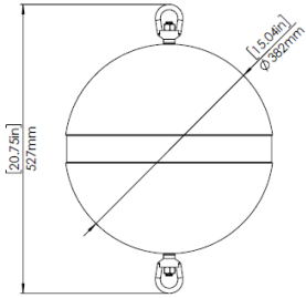
15" de Diámetro Modelo: SL-BF-15-S (Mostrado con extremos giratorios opcionales)
